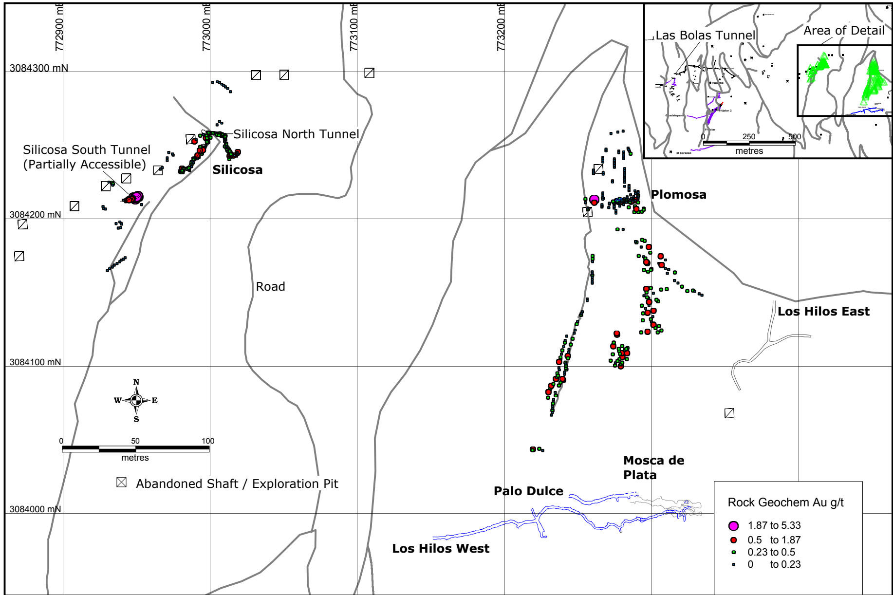
LAS BOLAS PROJECT CHANNEL-SAMPLES ROCK GEOCHEM Au g/t
